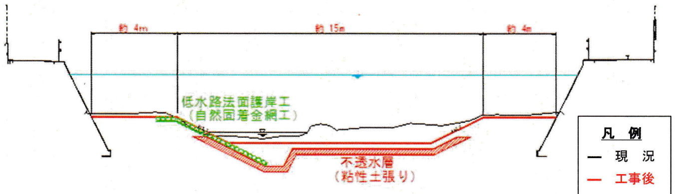
標準断面図
